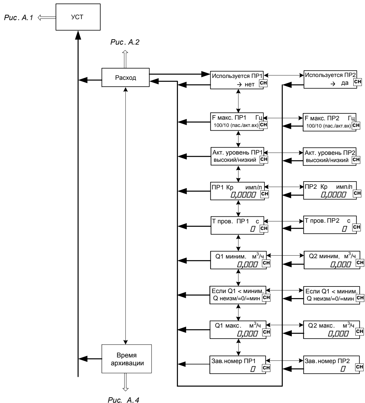
Рис.А.3. Меню «УСТ» и подменю «Расход».
