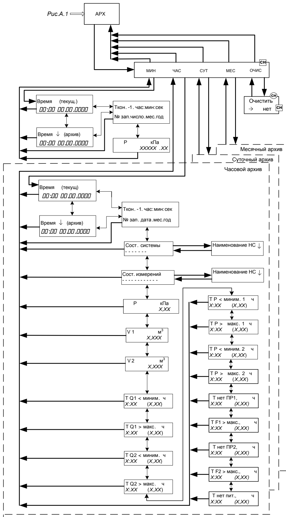
Рис.А.5. Меню «АРХ».
