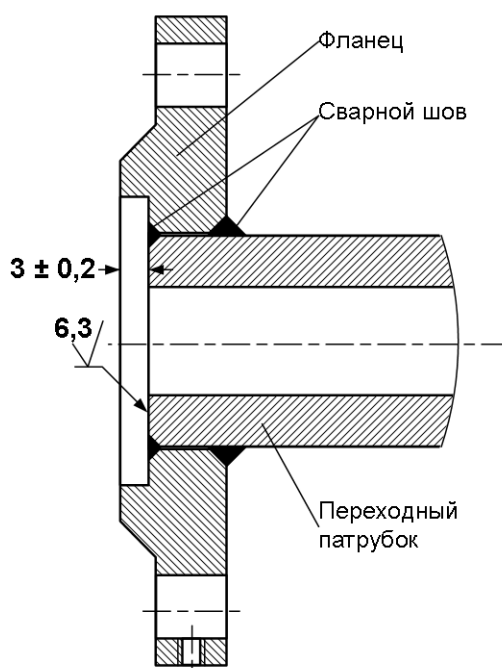
Рис.В.3. Вид и размеры переходных патрубков DN10, DN15.
