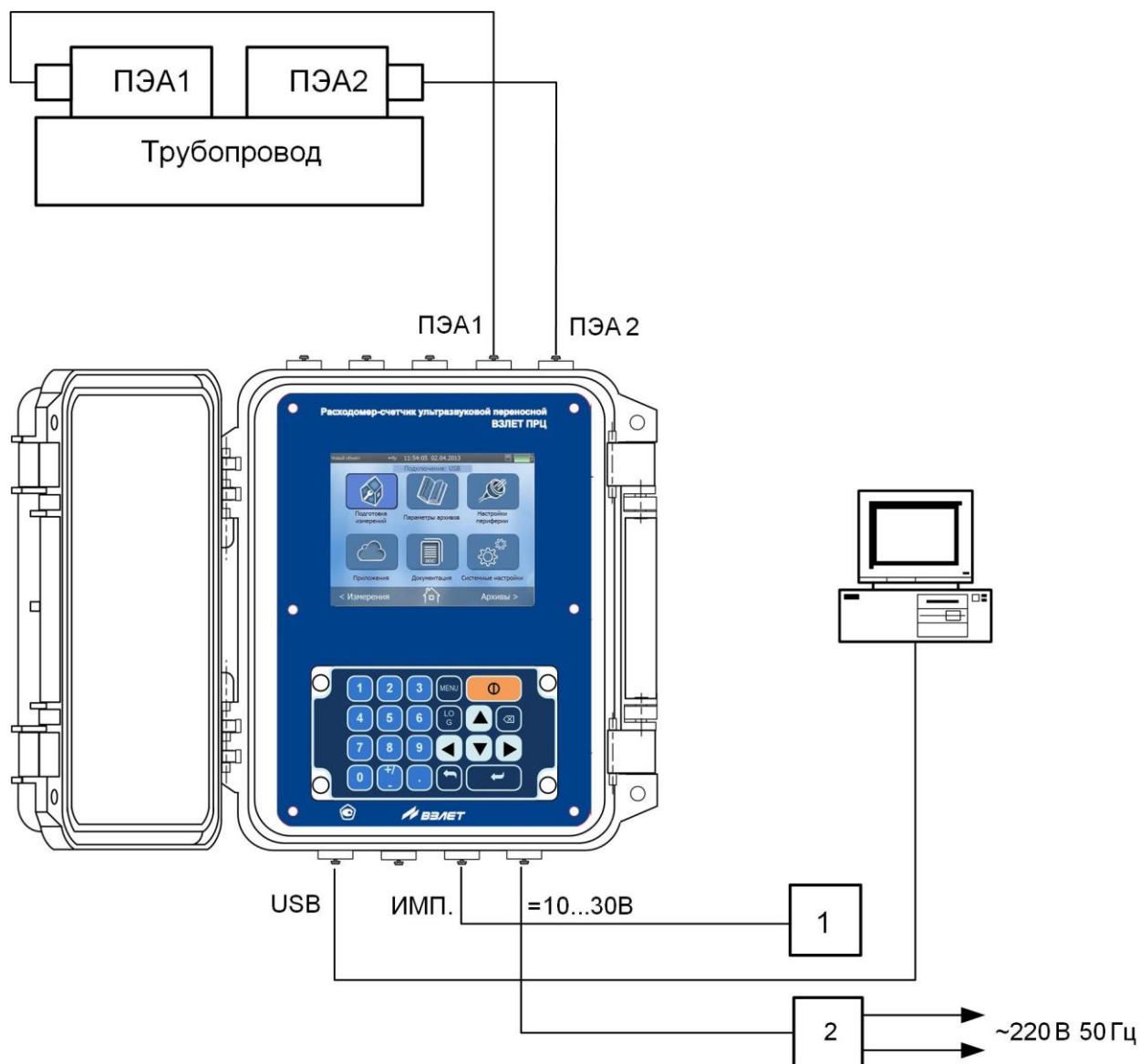
Рис.Г.1. Структурная схема поверки расходомера методом непосредственного сличения на поверочной установке.
