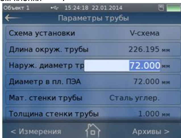
Рис.5. Пример индикации установки числовых значений параметра «Наруж. диаметр трубы» в окне «Параметры трубы».
