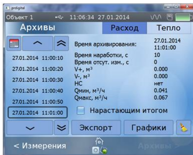
Рис.16. Отображение использования окон «Графики» и «Экспорт».
