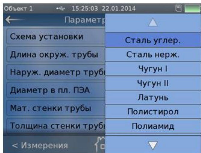
Рис.7. Пример индикации выбора списочных параметров в окне «Мат. стенки трубы» меню «Параметры трубы».
