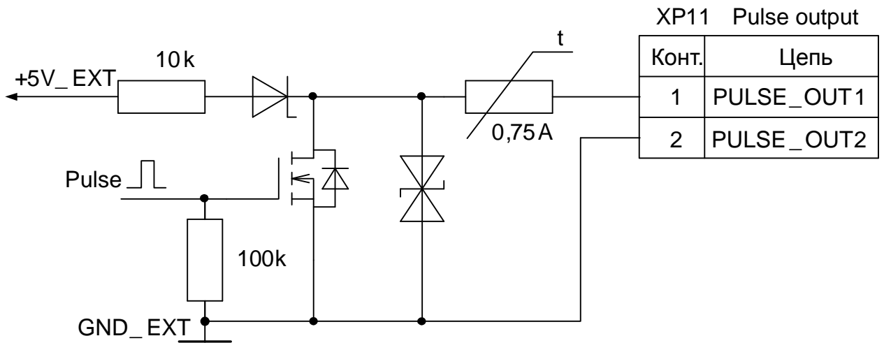
Рис.Б.1. Схема оконечного каскада универсального выхода.
