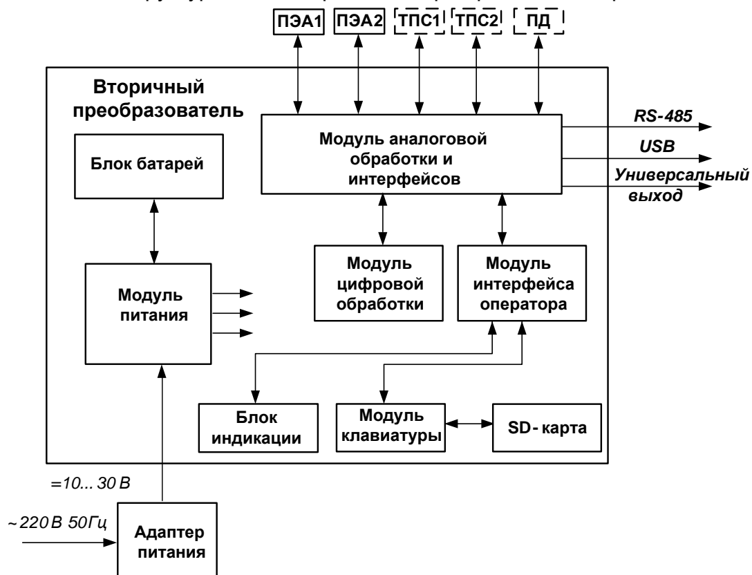
Рис.3. Структурная схема расходомера.
